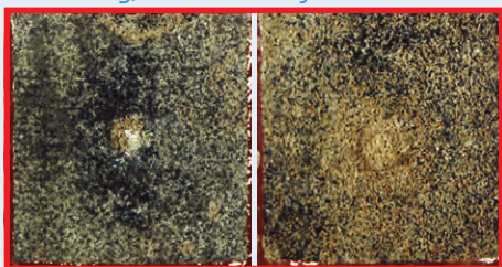
∇ ZnAl 600g/m 2 + Bitumen filler
